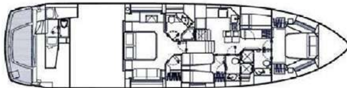
Planta baja
